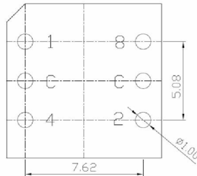
P.C.B. DIMENSION
