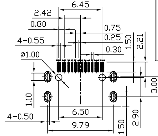
P.C.B LAYOUT
