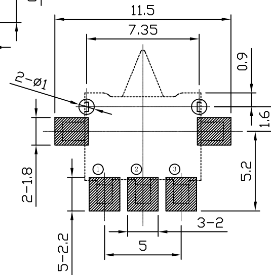
P.C.B LAYOUT
