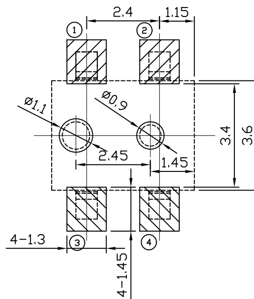
P.C.B LAYOUT
