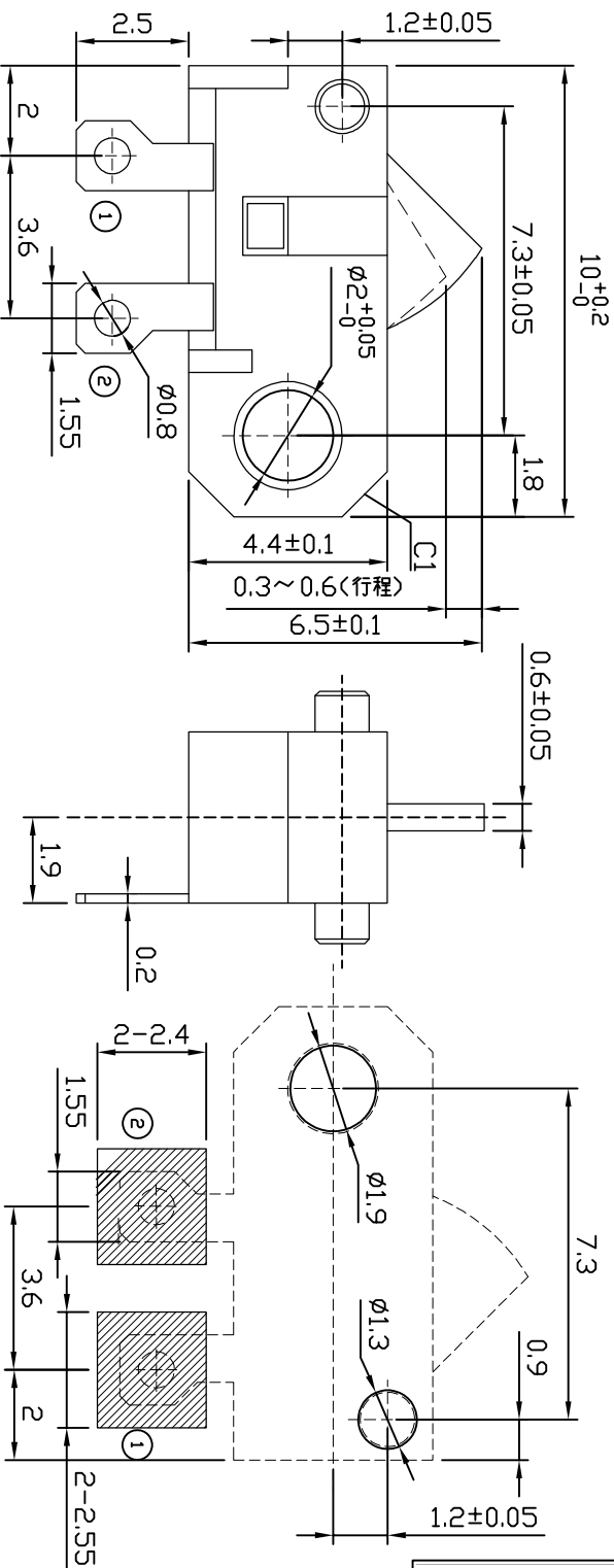
P.C.B LAYOUT
