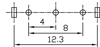
P.C.B LAYOUT
