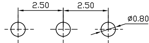
P.C.B LAYOUT
