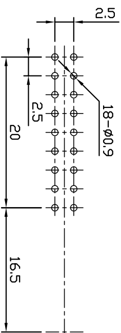
P.C.B LAYOUT
