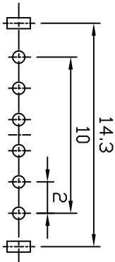
P.C.B LAYOUT
