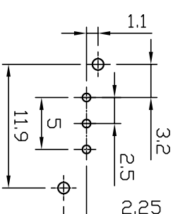
P.C.B LAYOUT
