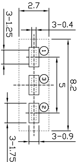
P.C.B LAYOUT
