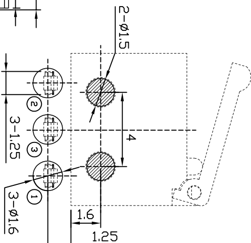
P.C.B LAYOUT
