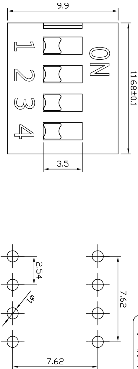
P.C.B LAYOUT
