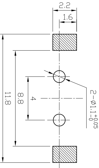
P.C.B LAYOUT
