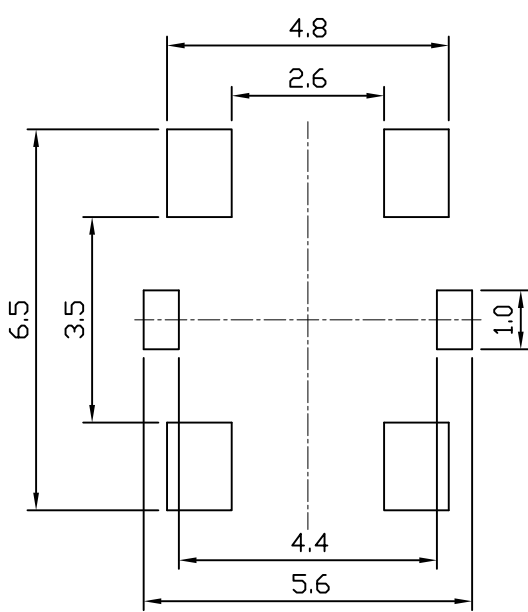
P.C.B LAYOUT
