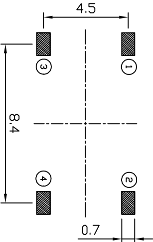
P.C.B LAYOUT
