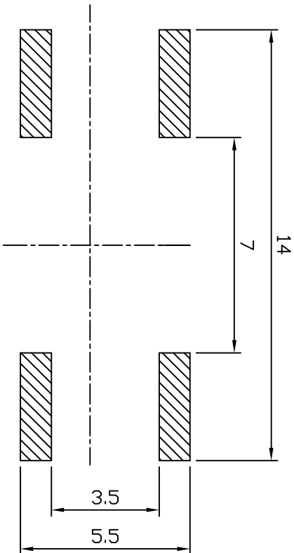
P.C.B LAYOUT
