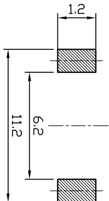
P.C.B LAYOUT
