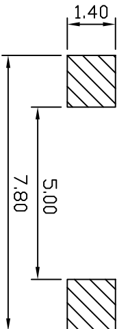
P.C.B LAYOUT
