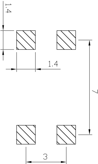
P.C.B LAYOUT
