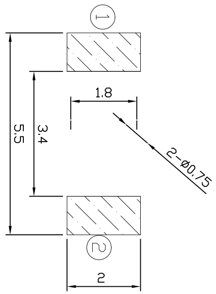
P.C.B. LAYOUT
