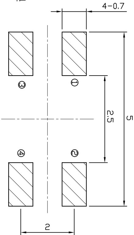
P.C.B LAYOUT
