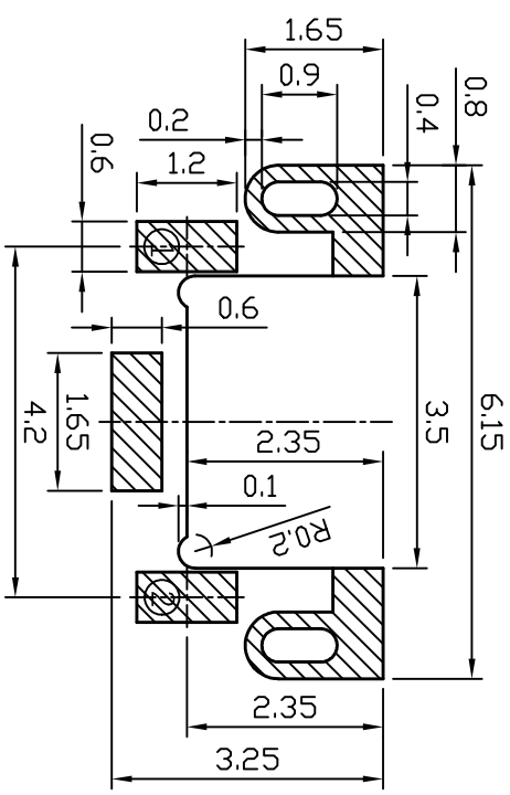
P.C.B LAYOUT
