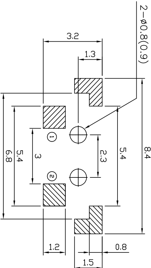
P.C.B LAYOUT
