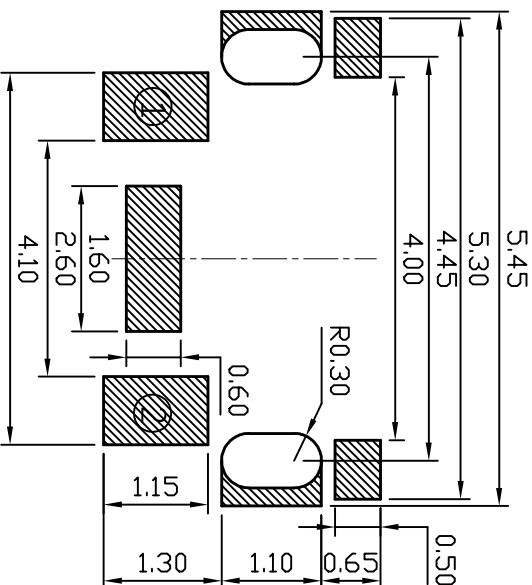
P.C.B LAYOUT
