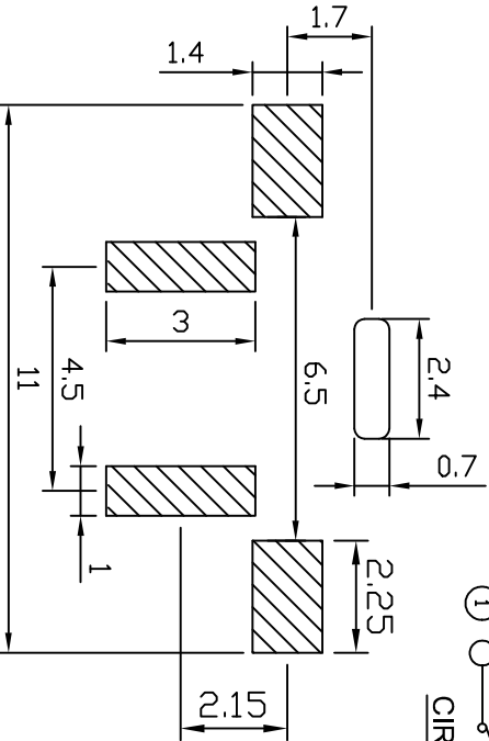
P.C.B LAYOUT
