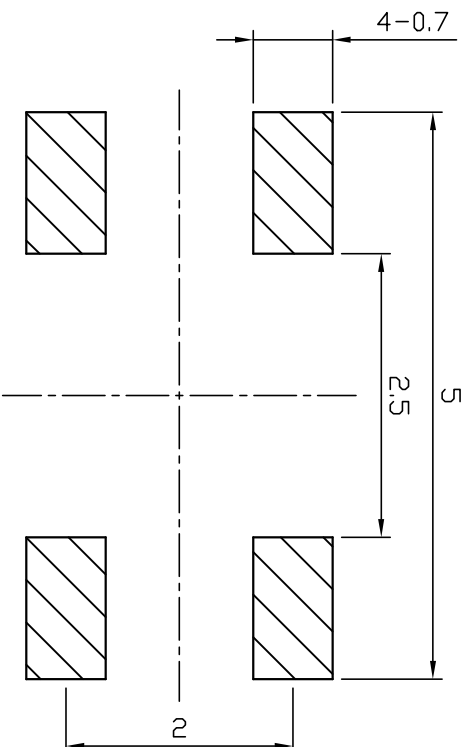
P.C.B LAYOUT
