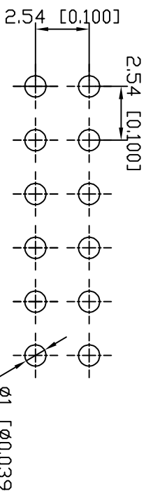
P.C.B LAYOUT
