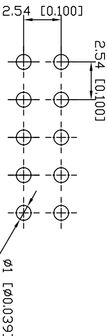
P.C.B LAYOUT
