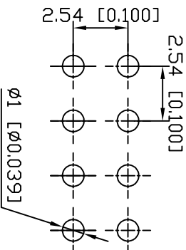
P.C.B LAYOUT
