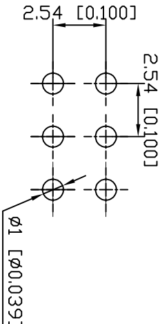
P.C.B LAYOUT
