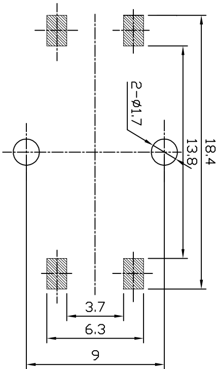
P.C.B LAYOUT
