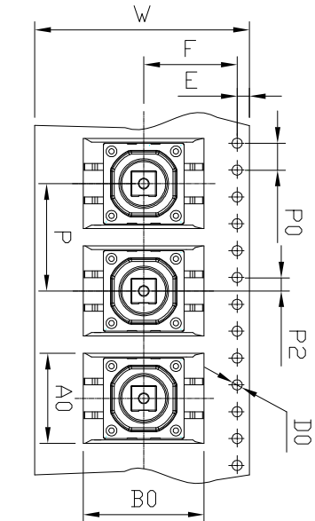
图1：成品载带
