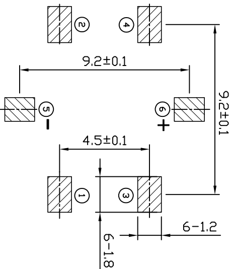
P.C.B LAYOUT
