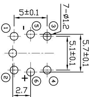
P.C.B LAYOUT
