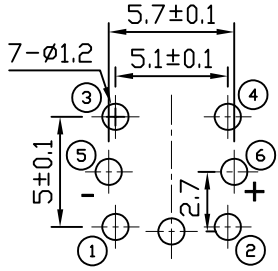
P.C.B LAYOUT
