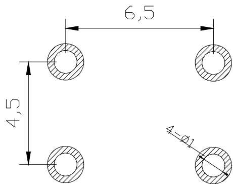
PCB. 焊接图
