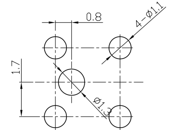
安装位置图
