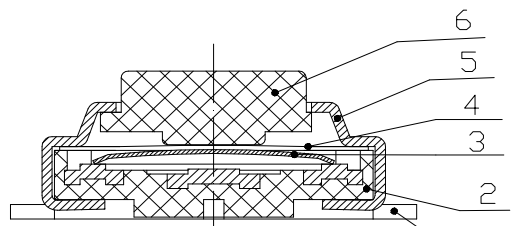
构造图
