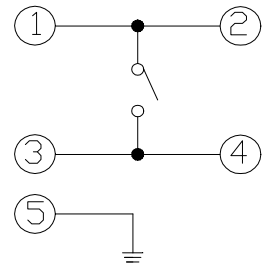
电气原理图
